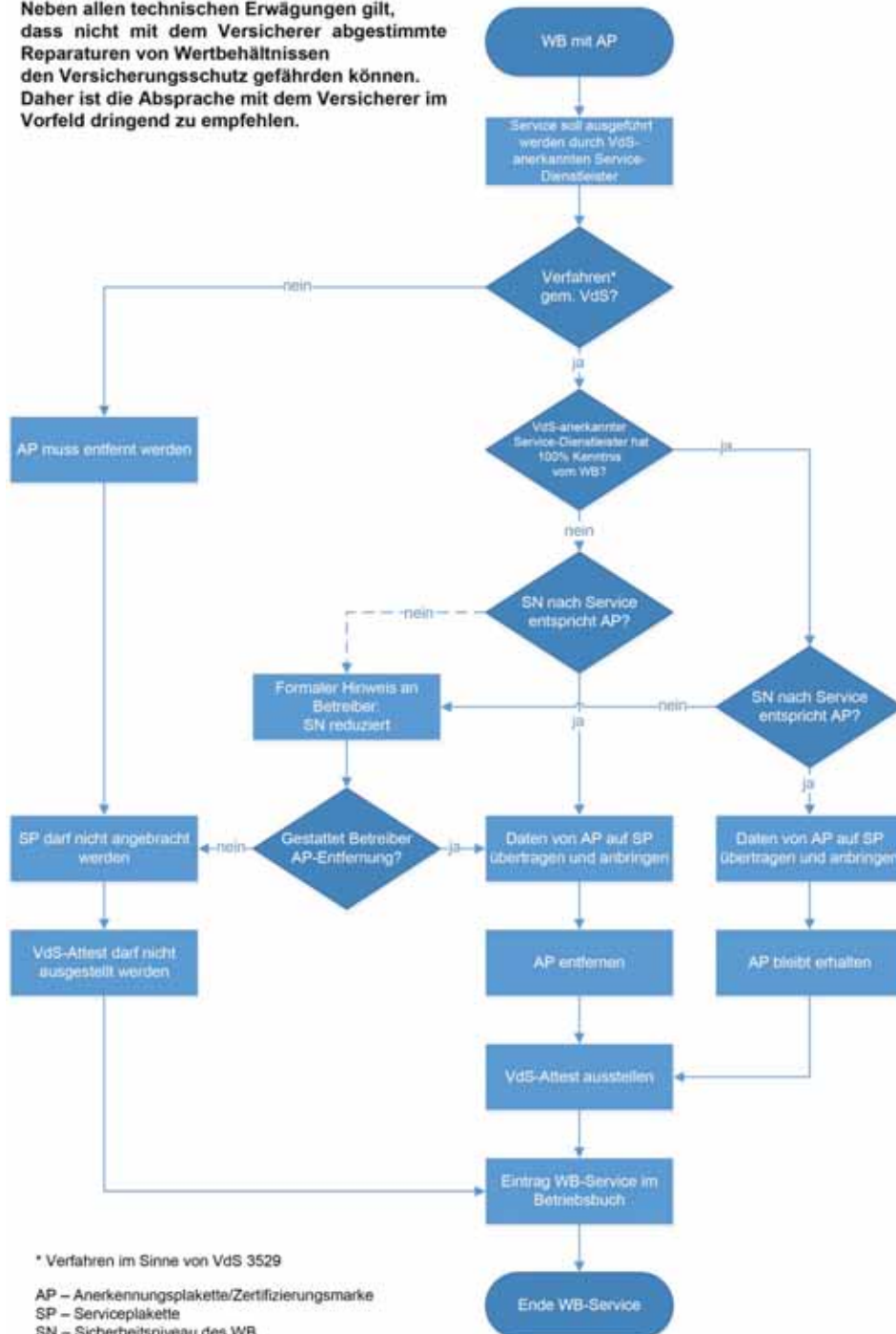
Bild 4: Ablauf von Servicemaßnahmen an WB für VdS-anerkannte Service-Dienstleister nach VdS 3529
