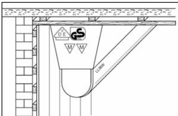
Bild 7: Leuchten müssen in ausreichendem Abstand zu brennbaren Flächen montiert werden.
