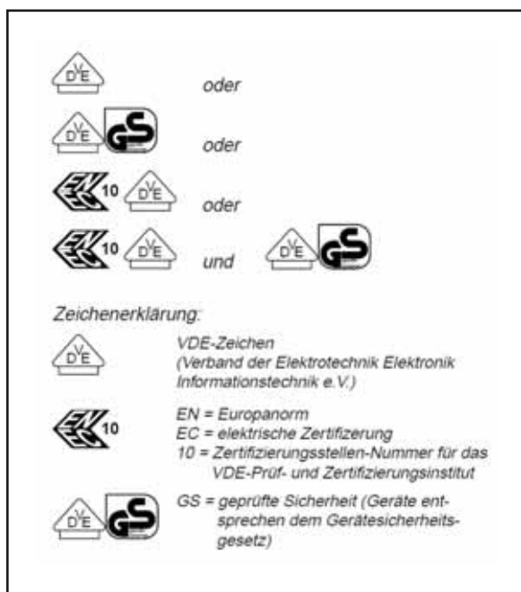
Bild 1: Prüfzeichen auf Leuchten.
