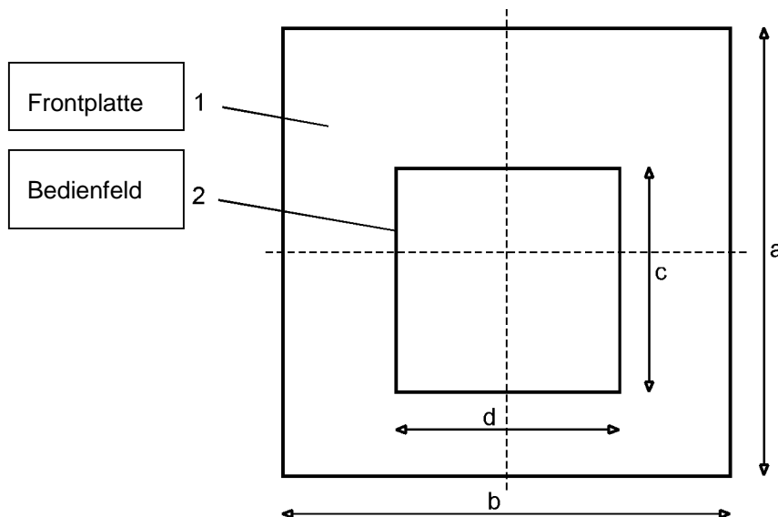
Abbildung 4.01: Abmessungen von Frontplatte und Bedienfeld
