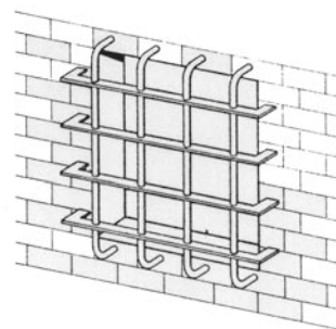
Bild 8-32: Auf die Wand aufgesetztes Gitter
