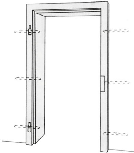
Bild 8-3: Türzarge
