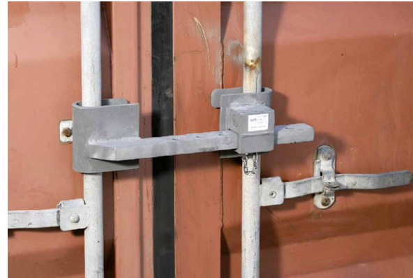
Abb. 5: Beispiel geeigneter Sicherungssysteme, Quelle: SUTainer Trans-Safety® GmbH
