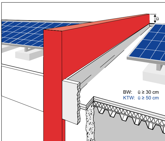
Bild 46: Erforderliche Erhöhung der Überdachung einer Brandwand
