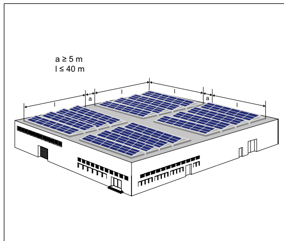
Bild 47: Unterteilung zusammenhängender Modulreihen und Modulaufstellflächen
