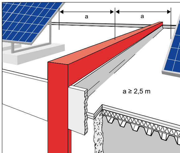
Bild 45: Erforderlicher Abstand zwischen der Überdachung einer Brandwand und Bauteilen der PV-Anlagen auf dem Dach, z. B. PV-Module oder Wechselrichter
