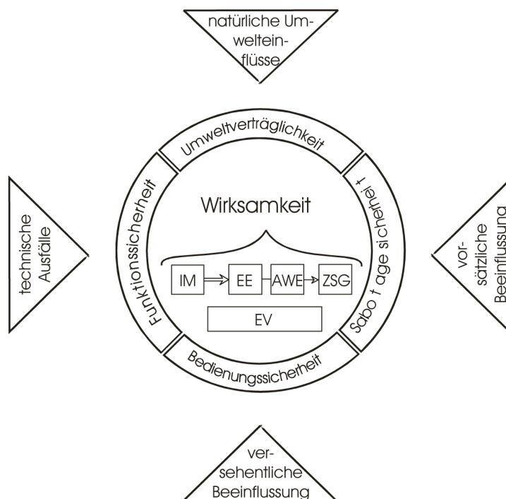
Bild 1.01: Schutzfunktionen einer ZKA
