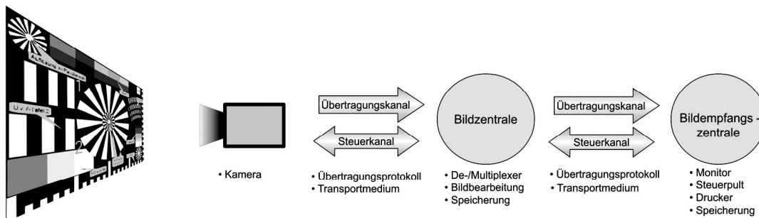
Bild 7.01 : Schematischer Prüfaufbau
