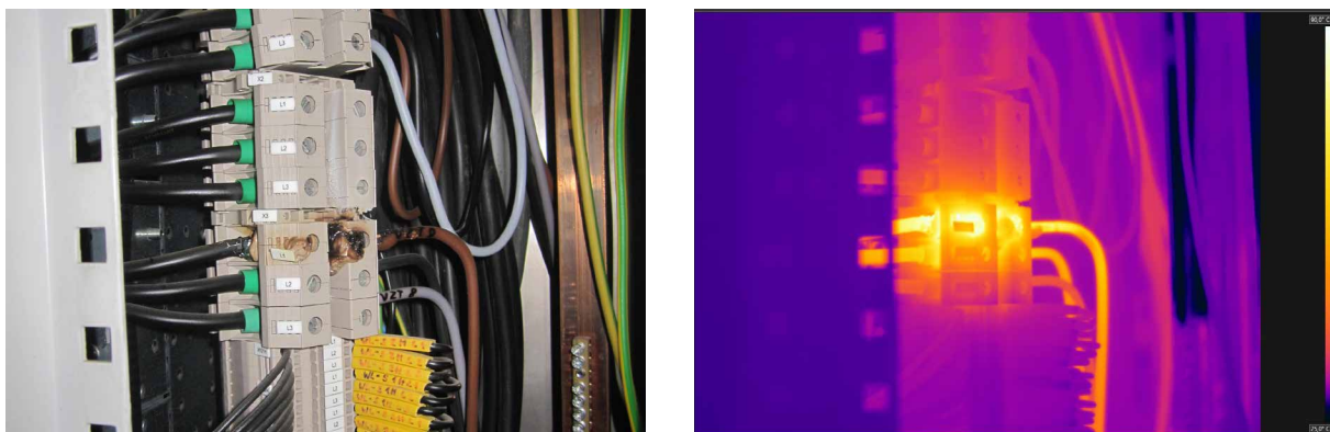
Klemmverbindung (Klemme L1 bei X3) Quelle: Lutz Erbe, VGH
