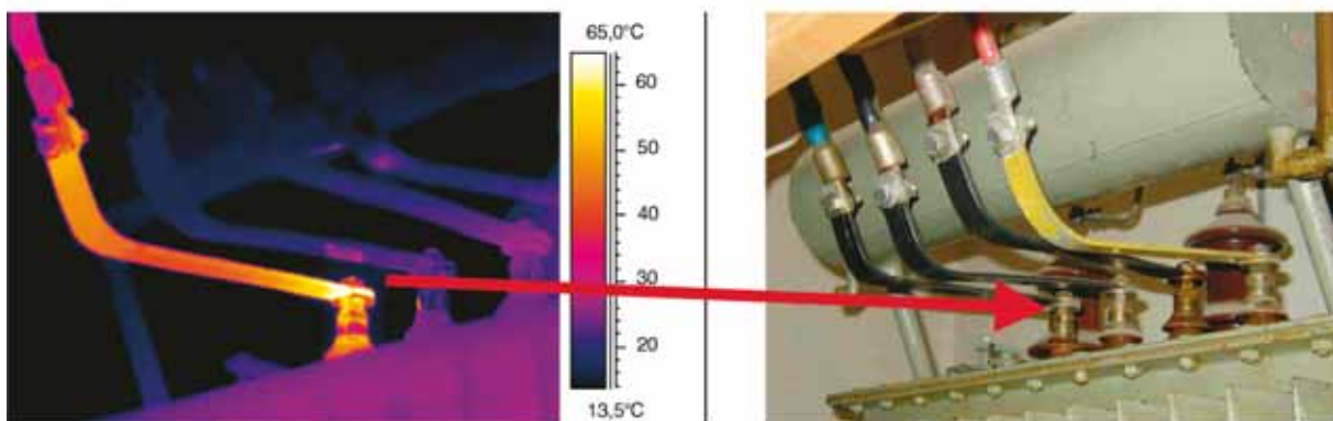
Defekte Schraubverbindung
