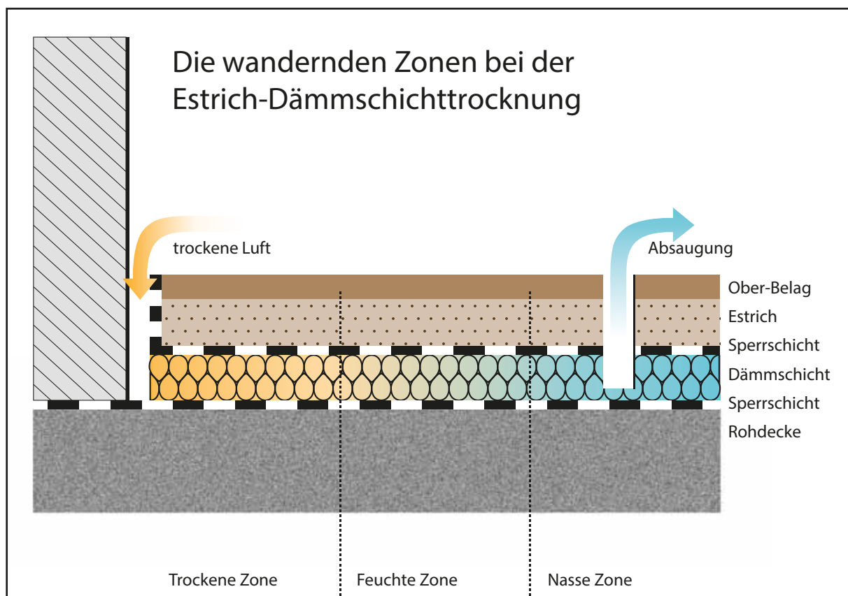
Abbildung: Die wandernden Zonen bei der Estrich-Dämmschichttrocknung. Schimmelpilzwachstum kann nur in der relativ schmalen feuchten Zone stattfinden. Bei Einhaltung der Regel-trocknungszeiten (siehe Anhang A7) kann kein Schimmelpilzwachstum entstehen.
