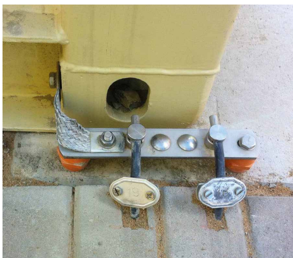
Bild 20: Einbindung von Anlagenteilen in den vermaschten Potentialausgleich
