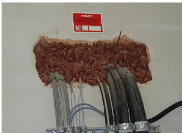
Bild 25: Bauaufsichtlich zugelassene Kabeldurchführung
