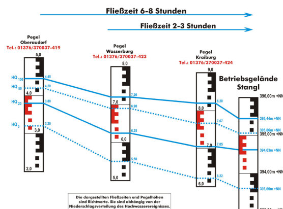
Abb. 8-7: Pegelbezugsdiagramm Stangl AG (Quelle: Sönnichsen&Weinert)
