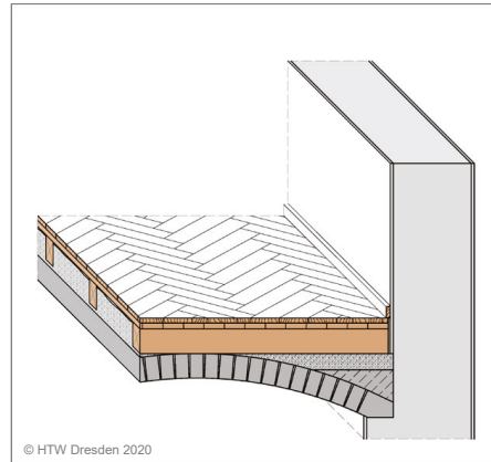
Kappendecke mit flacher Wölblinie
