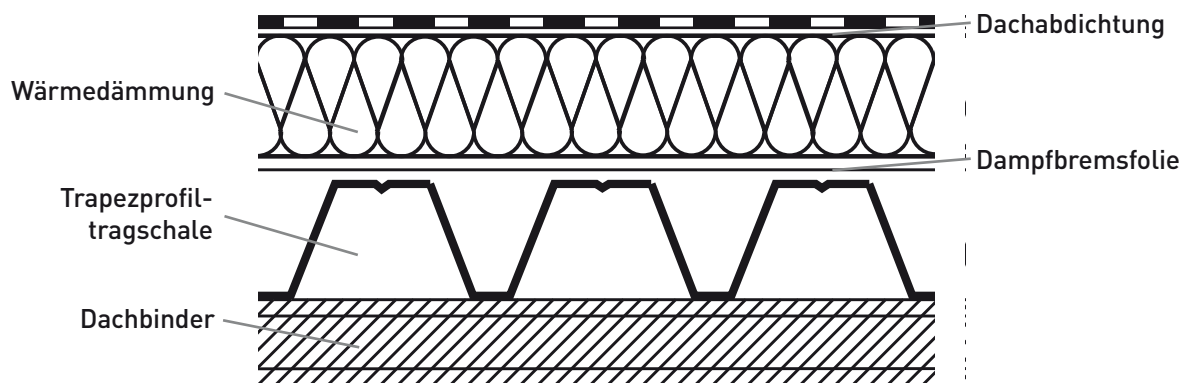
Bild 2: Beispielhafter Aufbau eines flachen bzw. flach geneigten Daches
